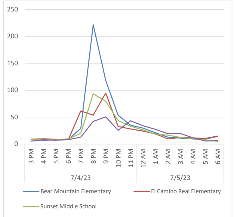
Promedio horario de PM2.5 el 4 de julio
