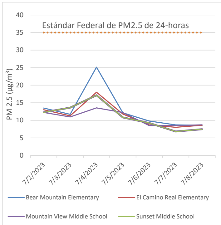
Promedio semanal de PM2.5 en períodos de 24 horas
