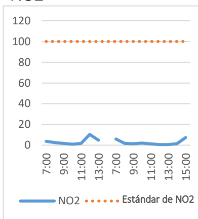
NO2
