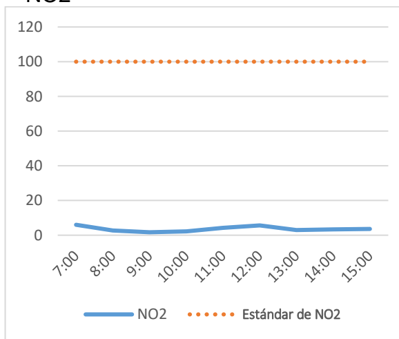
NO2
