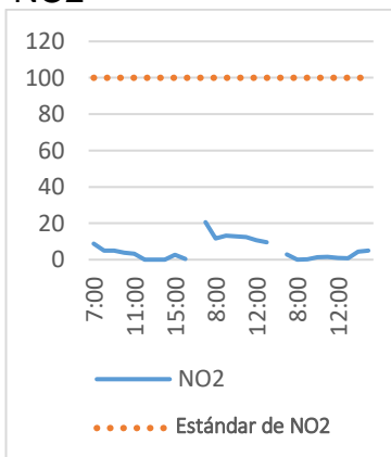
NO2
